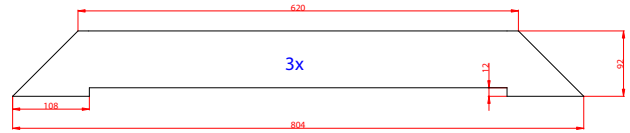
DISTANZST-CK OBEN
