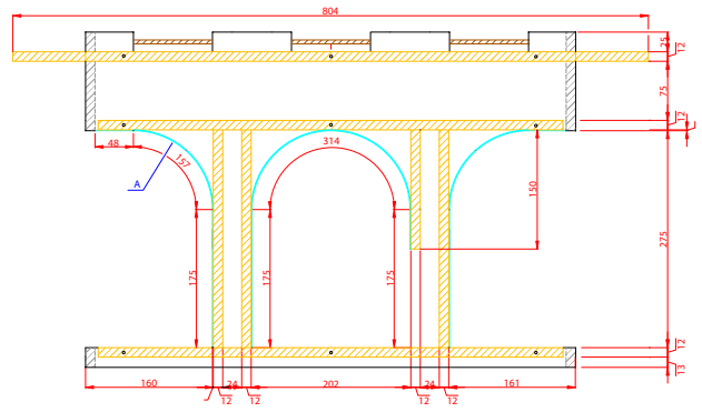
INNENWAND
